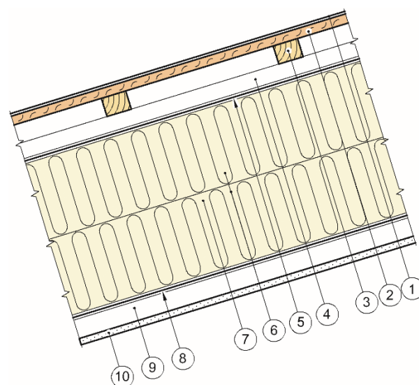
Vertikalsnitt
