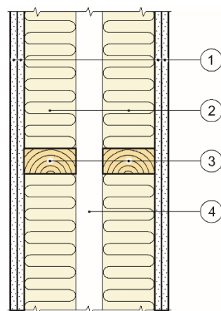
Horizontalsnitt
