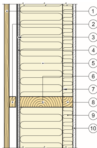
Horizontalsnitt
