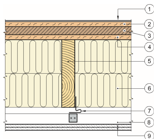
Vertikalsnitt
