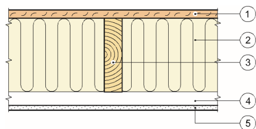
Vertikalsnitt
