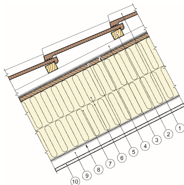
Vertikalsnitt
