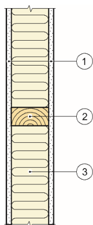
Horizontalsnitt
