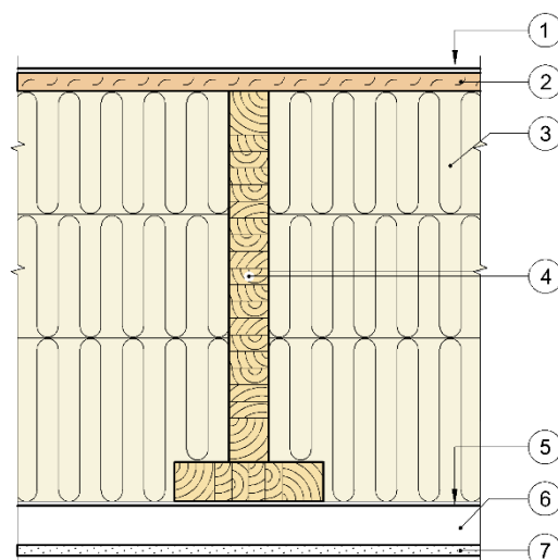
Fig. 8 Prinsipiell oppbygning av flate kompakte tretak med fuktadaptiv dampsperre med heltrebbjelker.
