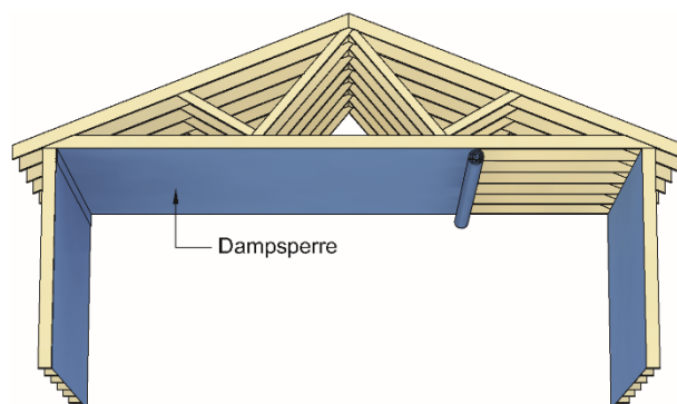
Fig. 1 Glava Dampsperre monteret i yttervegg og mot kaldt loftsrom
