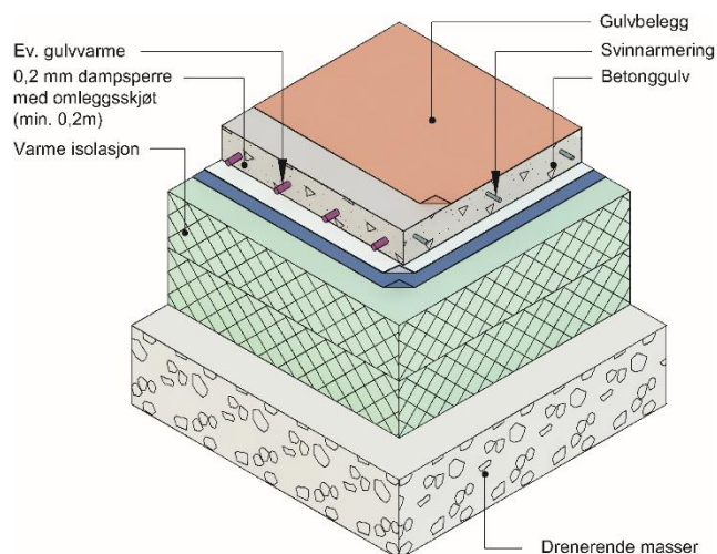
Fig. 3 Siga Dampsperre monteret i betonggolv på grunnen
