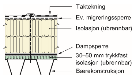
Fig. 2 Siga Dampsperre monteret i kompakt takkonstruksjon
