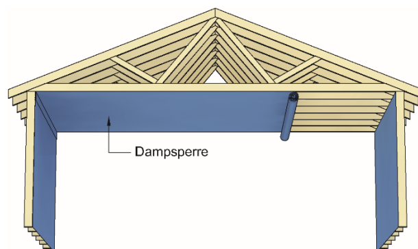
Fig. 1 Siga Dampsperre monteret i yttervegger og mot kaldt loftsrom
