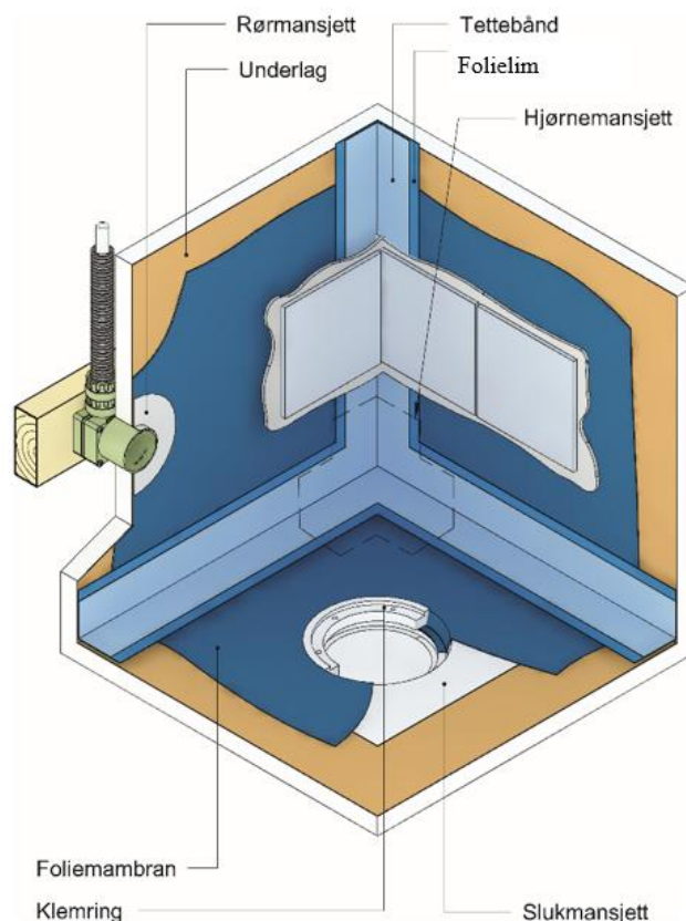
Fig. 1. Oppbygning av Sopro membransystem
