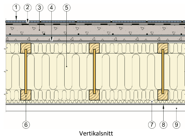
Fig. 6 Prinsipiell oppbygning av etasjeskiller over fundament
