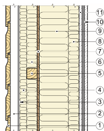
Vertikalsnitt
