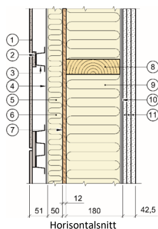
Fig. 2 Prinsipiell oppbygning av yttervegger med horisontal trekledning
