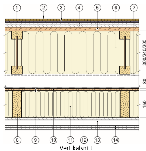
Fig. 9 Prinsipiell oppbygning av standard etasjeskiller mellom moduler. Øvre del er gulvkonstruksjon i øvre etasje, nedre del er tak/himlingskonstruksjon i nedre modul. Bjelkeavstand i henhold til spesifikk dimensjonering
