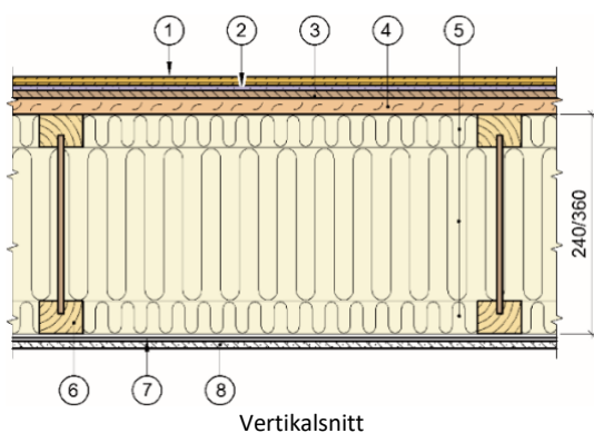
Fig. 7 Prinsipiell oppbygning av skillevegger mellom moduler
