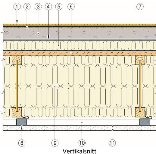
Fig. 11 Prinsipiell oppbygning av etasjeskiller i badetrom over fundament. Bjelke dimensjon og bjelkeavstand i henhold til spesifikk dimensjonering. I etasjeskiller mellom moduler erstattes vindspærren med stålnetting
