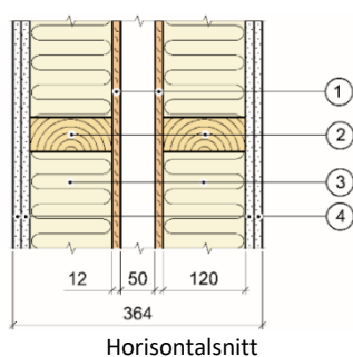
Fig. 6 Prinsipiell oppbygning av innervegger
