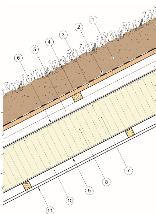
Fig. 7 Prinsipiell oppbygning av skrå tak med opplettet tekning. Elementene leveres fra fabrikk med sperrer, undertak, sløyfer og steinkleter.
