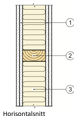
Horisontalsnitt
