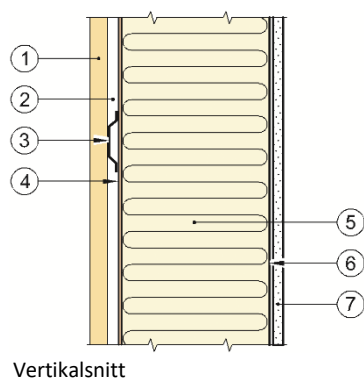
Vertikalsnitt
