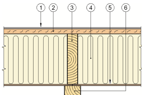
Vertikalsnitt
