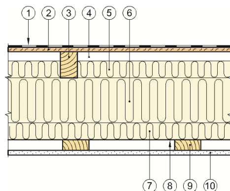
Vertikalsnitt
